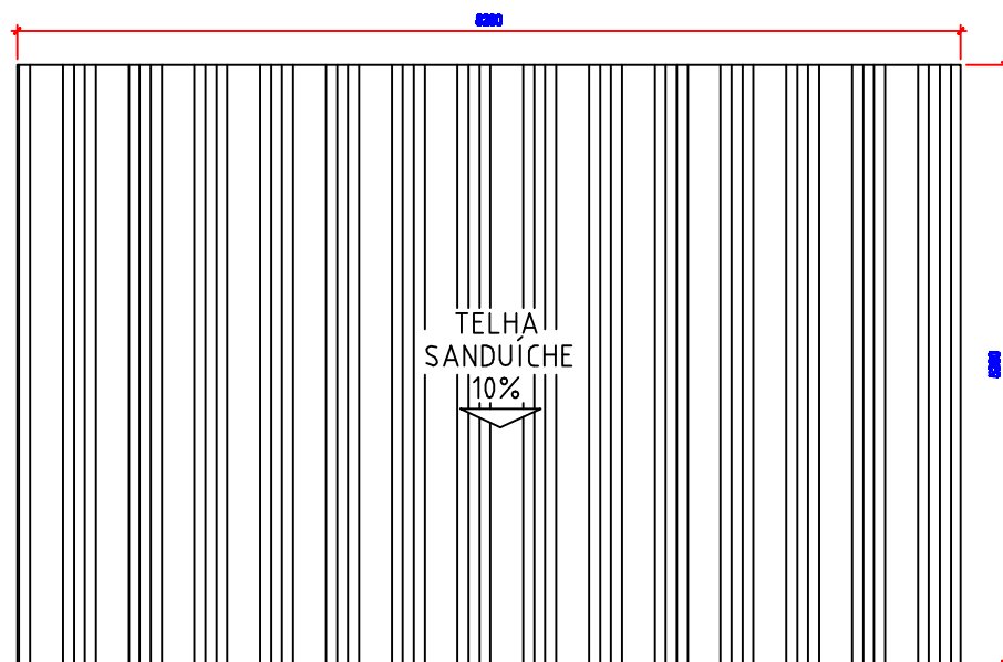
PLANTA DE COBERTURA Esc: 1/50
